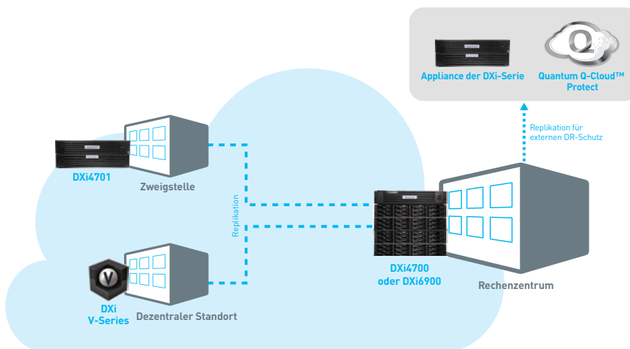
Abbildung 1 – Replikation von Backup-Daten für automatischen DR-Schutz
